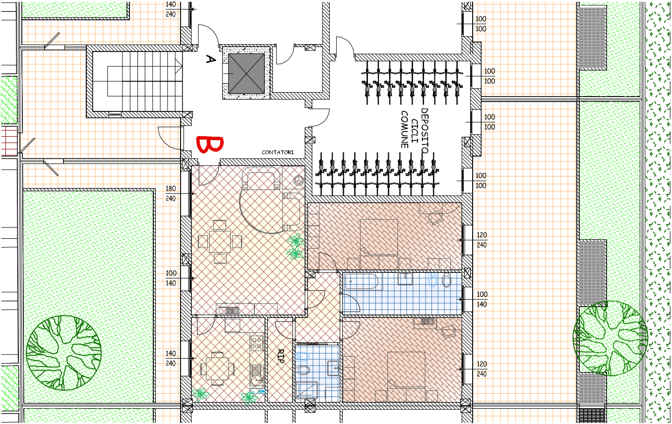
Pianta Arredata
