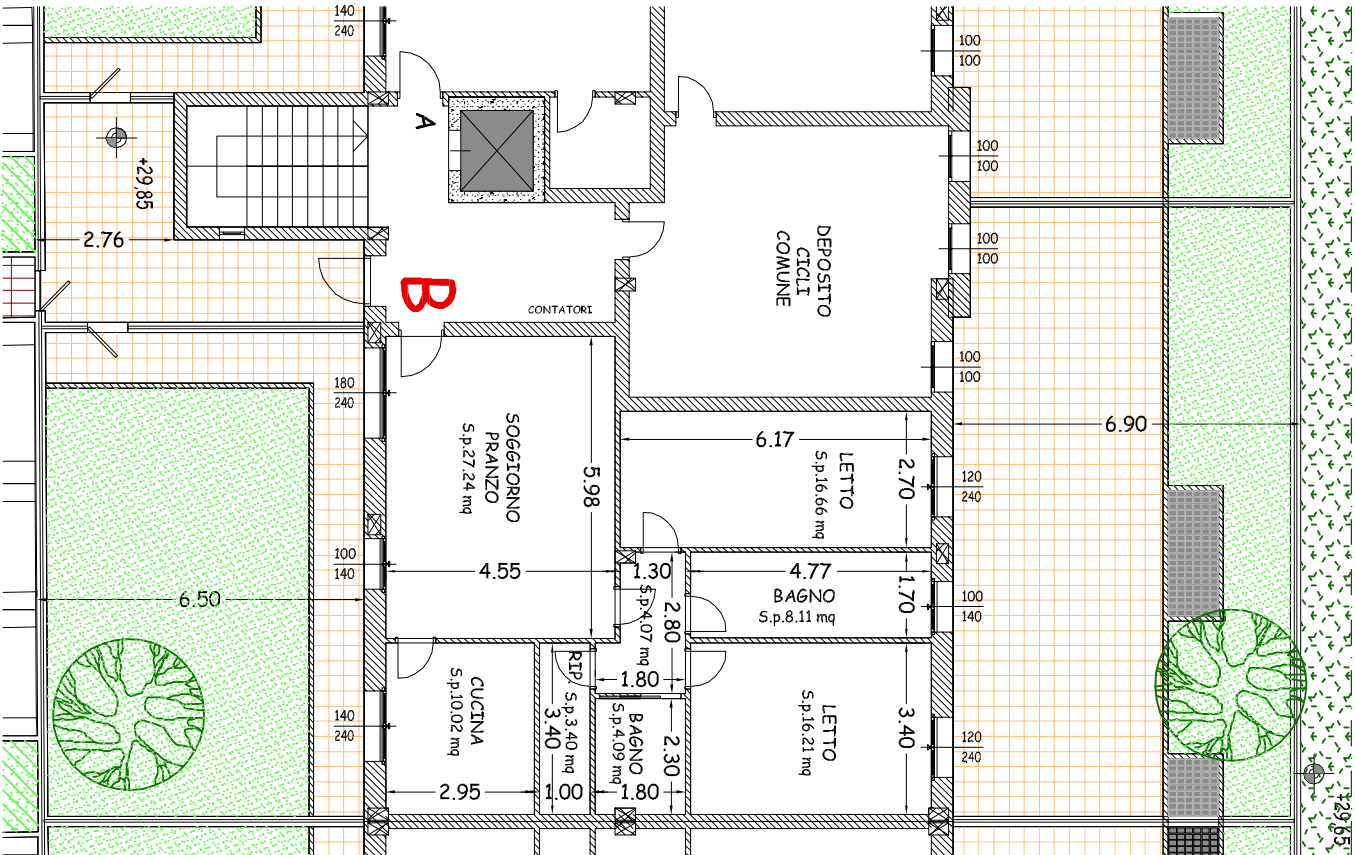
Pianta Quotata
